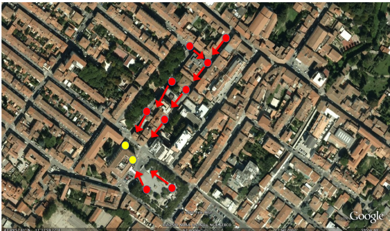
Figura n.4 – Hot spot Centro: posizionamento delle varie celle Wi-Fi e rete di backbone
